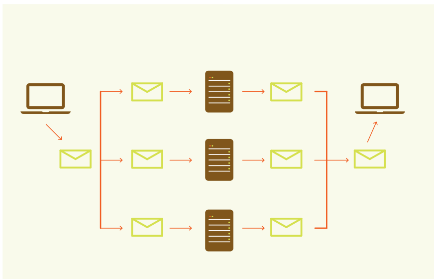
Protocolo TCP/IP
